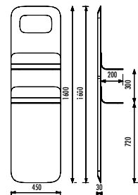
FL1045.03 Foglia Duvar Ünitesi Rafı Kumlmalı Led Aydınlatmalı (450x1600x30 mm) (GxYxD)
