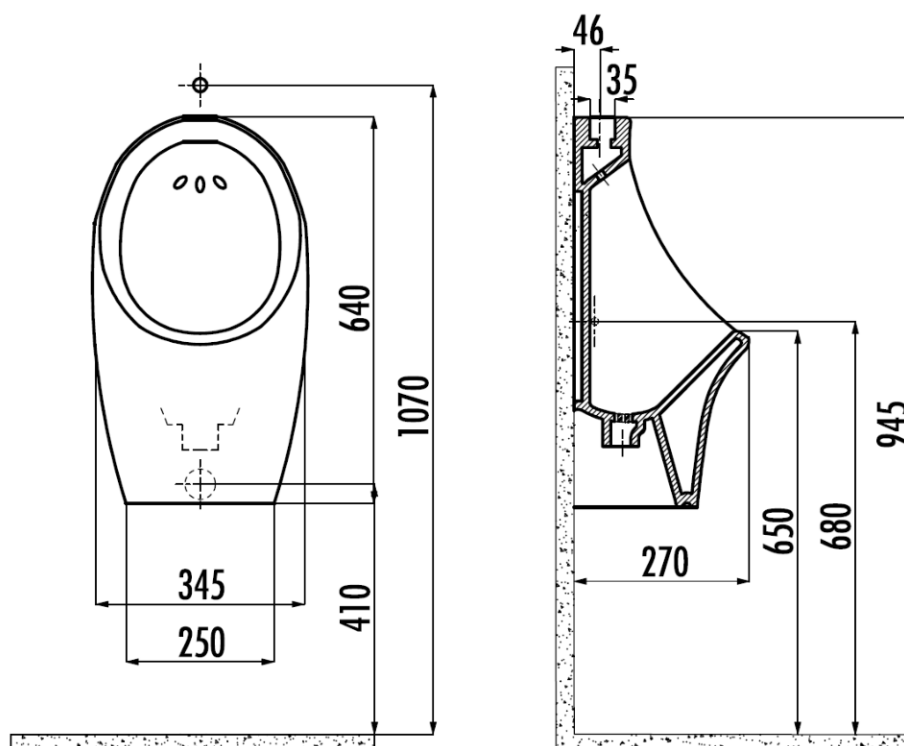
Схема монтажа писсуара (верхняя подводка воды)
