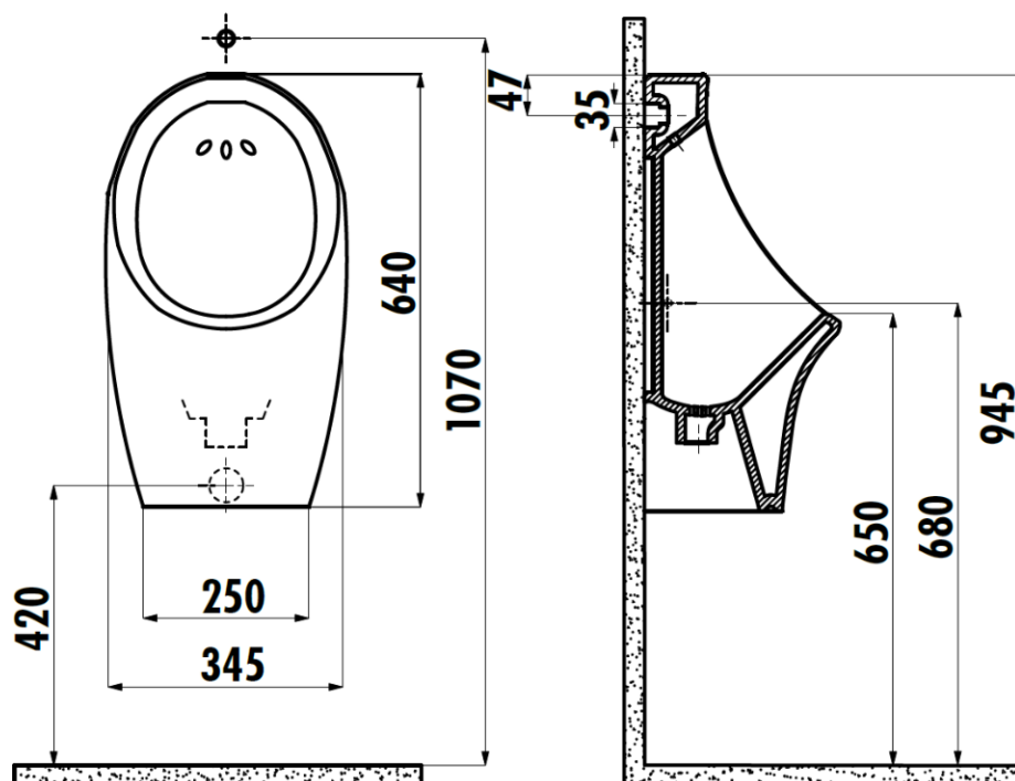
Схема монтажа писсуара (задняя подводка воды)
