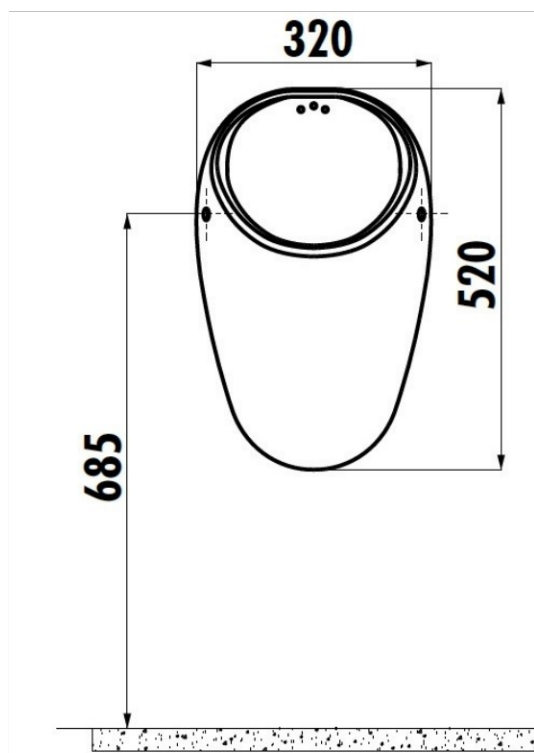
Схема монтажа писсуара (верхняя подводка воды)
