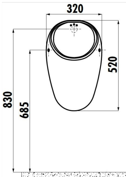
Схема монтажа писсуара (задняя подводка воды)
