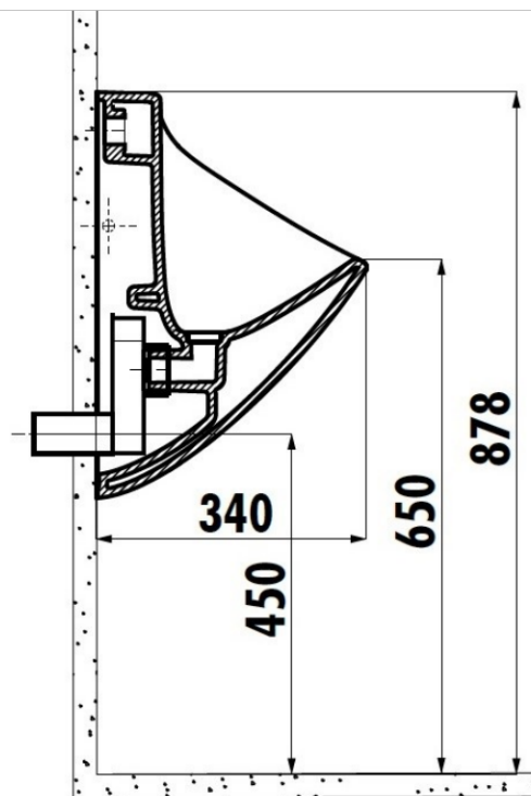
Схема монтажа писсуара (задняя подводка воды)
