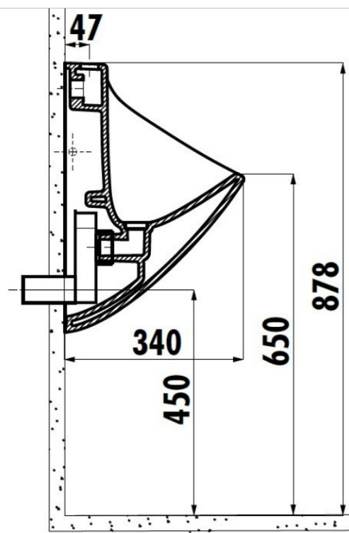
Схема монтажа писсуара (верхняя подводка воды)
