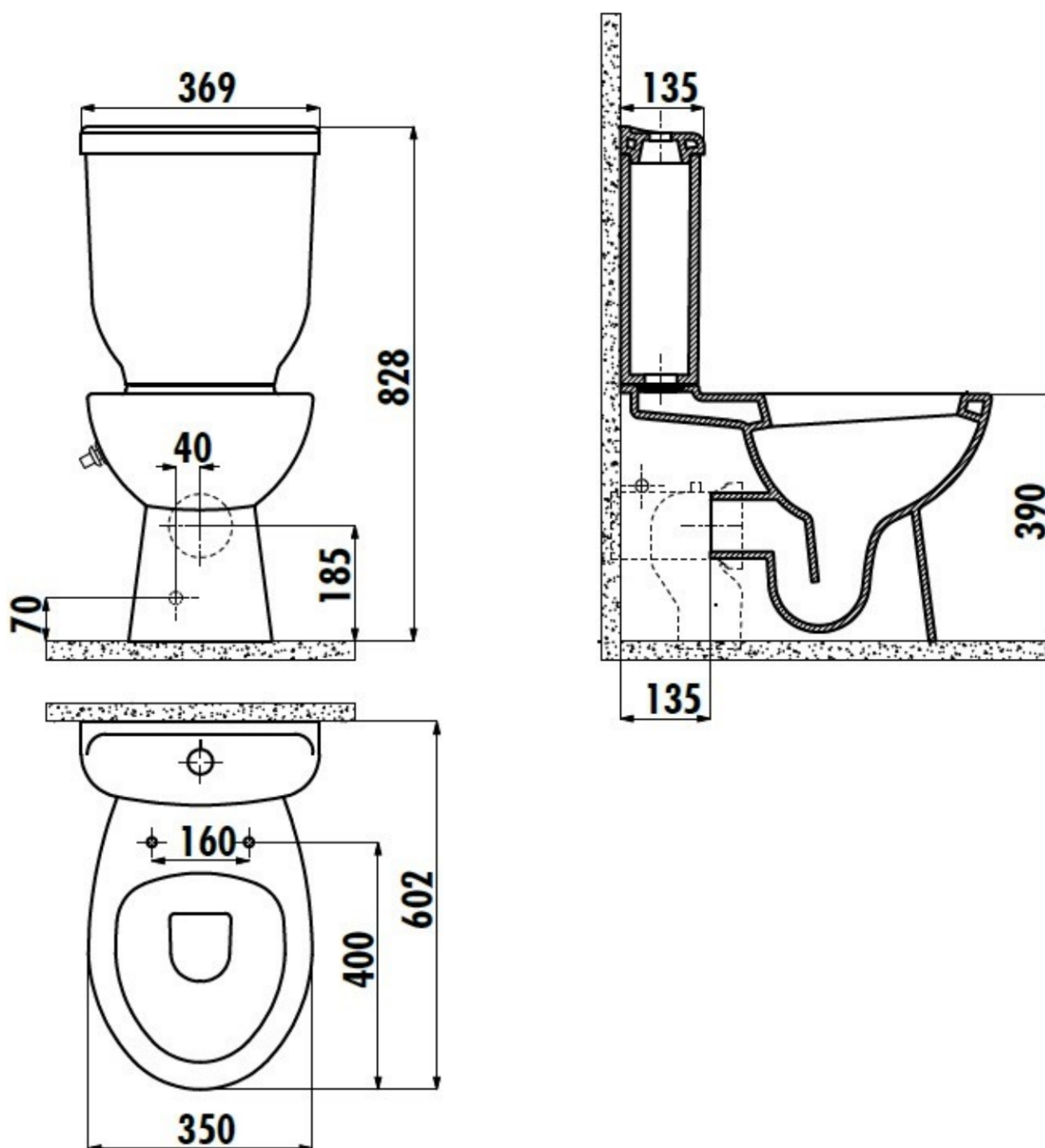
Схема монтажа унитаза (со встроенным краном)
