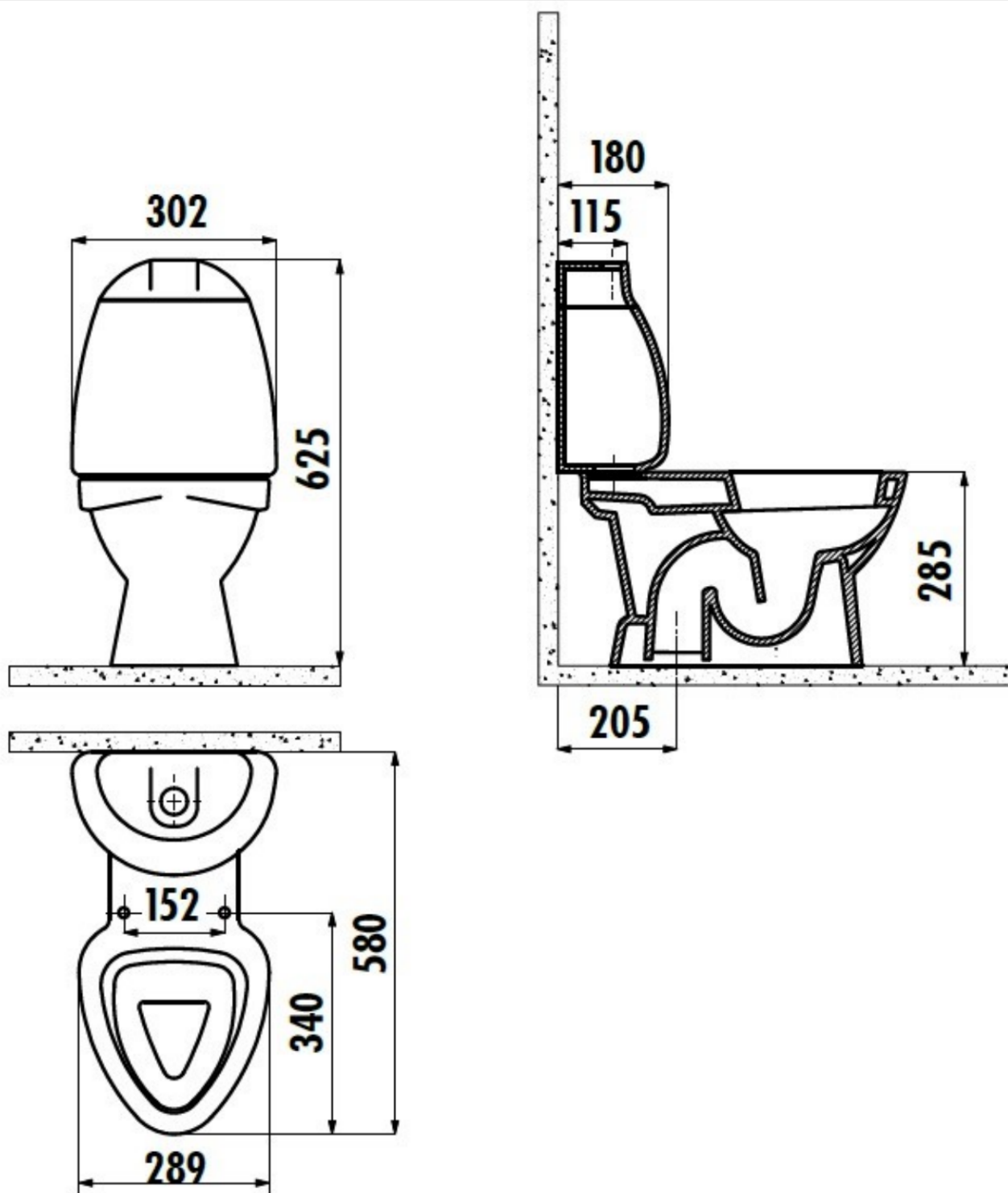
Схема монтажа унитаза
